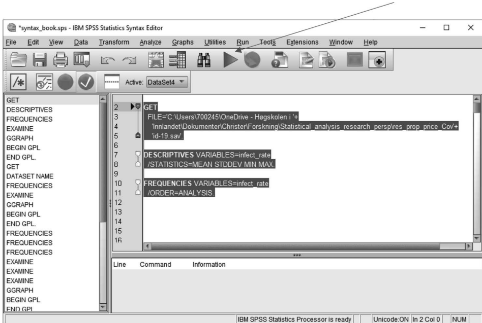
SPSS-output 2.5 An example of a short SPSS syntax-file.
