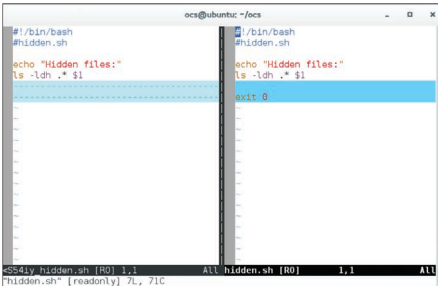
Figure 15-9 git difftool using vimdiff
